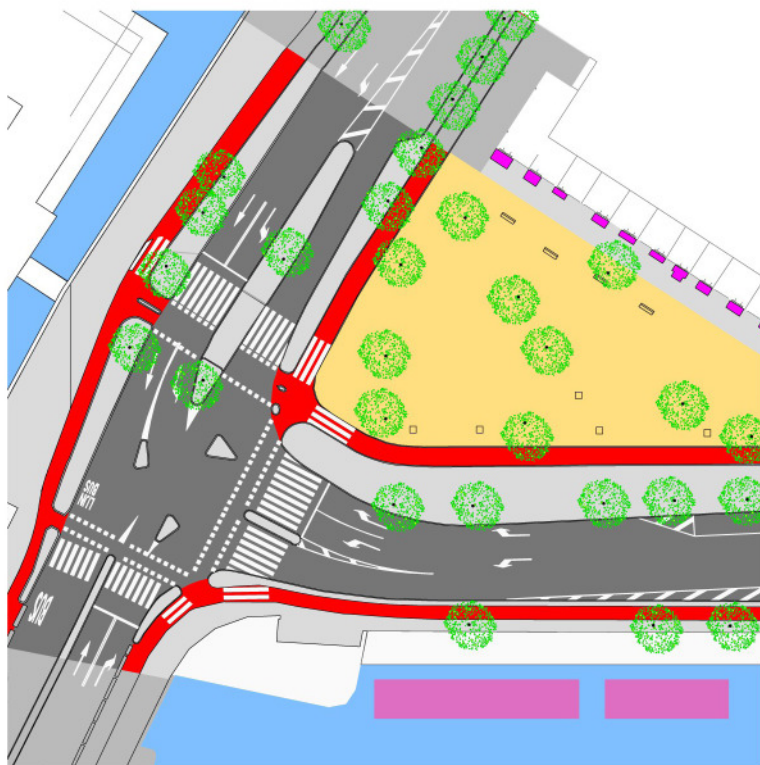
0. Uitsnede plattegrond Eilandenboulevard Kattenburgerplein - Bestaande situatie 0 5 10 15 20 25 50m
