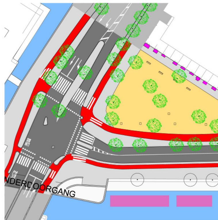
1. Uitsnede plattegrond Eilandenboulevard Kattenburgerplein - Variant 1 0 5 10 15 20 25 50m
