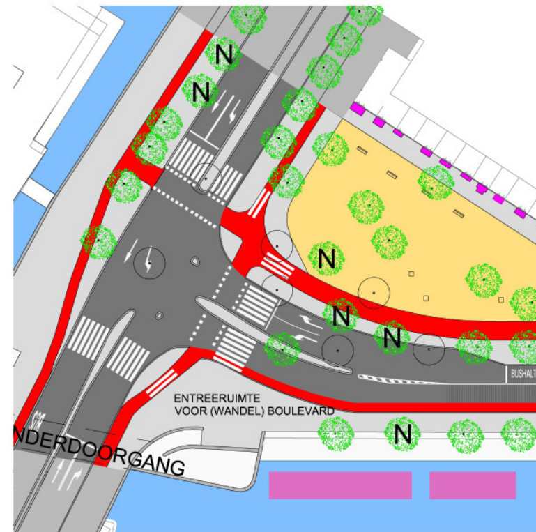
3. Uitsnede plattegrond Eilandenboulevard Kattenburgerplein - Variant 3 0 5 10 15 20 25 50m
